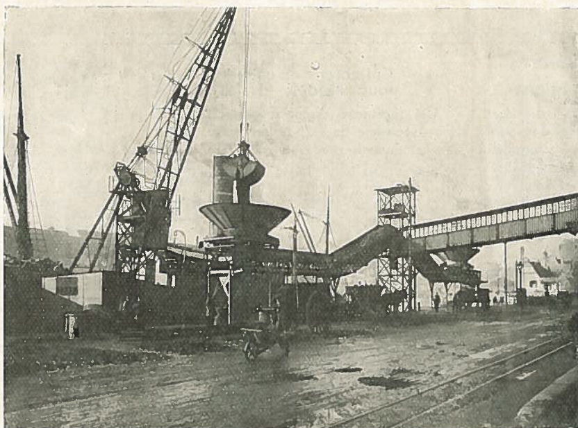
Autre aspect du Transbordeur Combiné.
