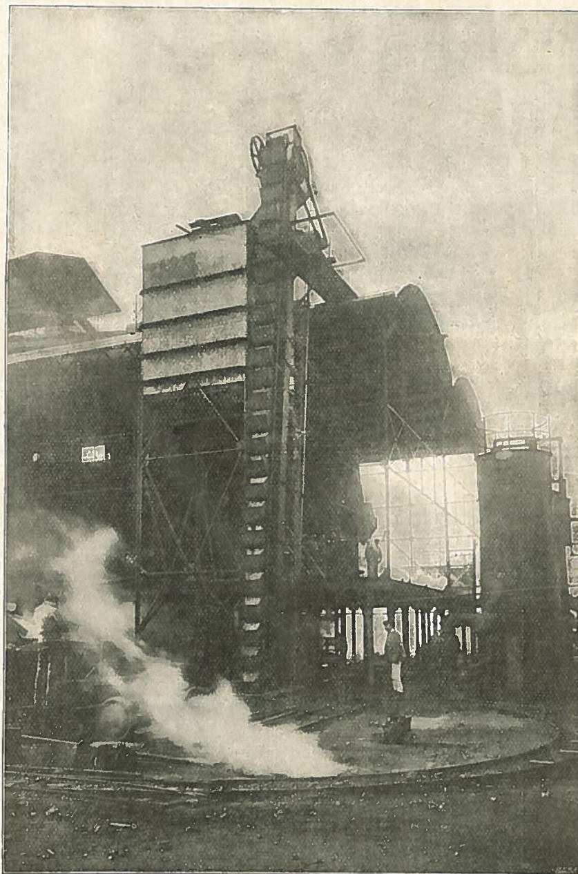
Élévateur incliné à double chaîne.
