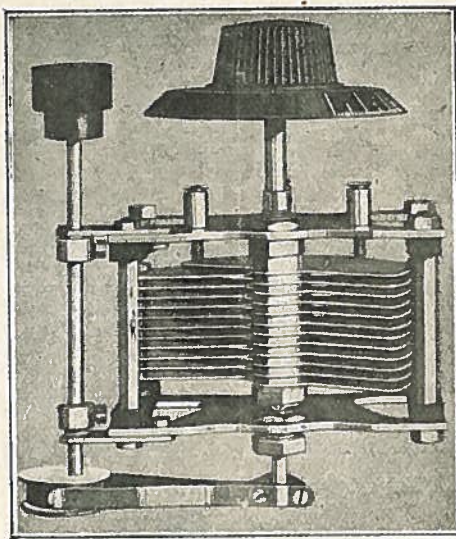
Condensateur variable. Modèle perfectionné à avance micrométrique.
