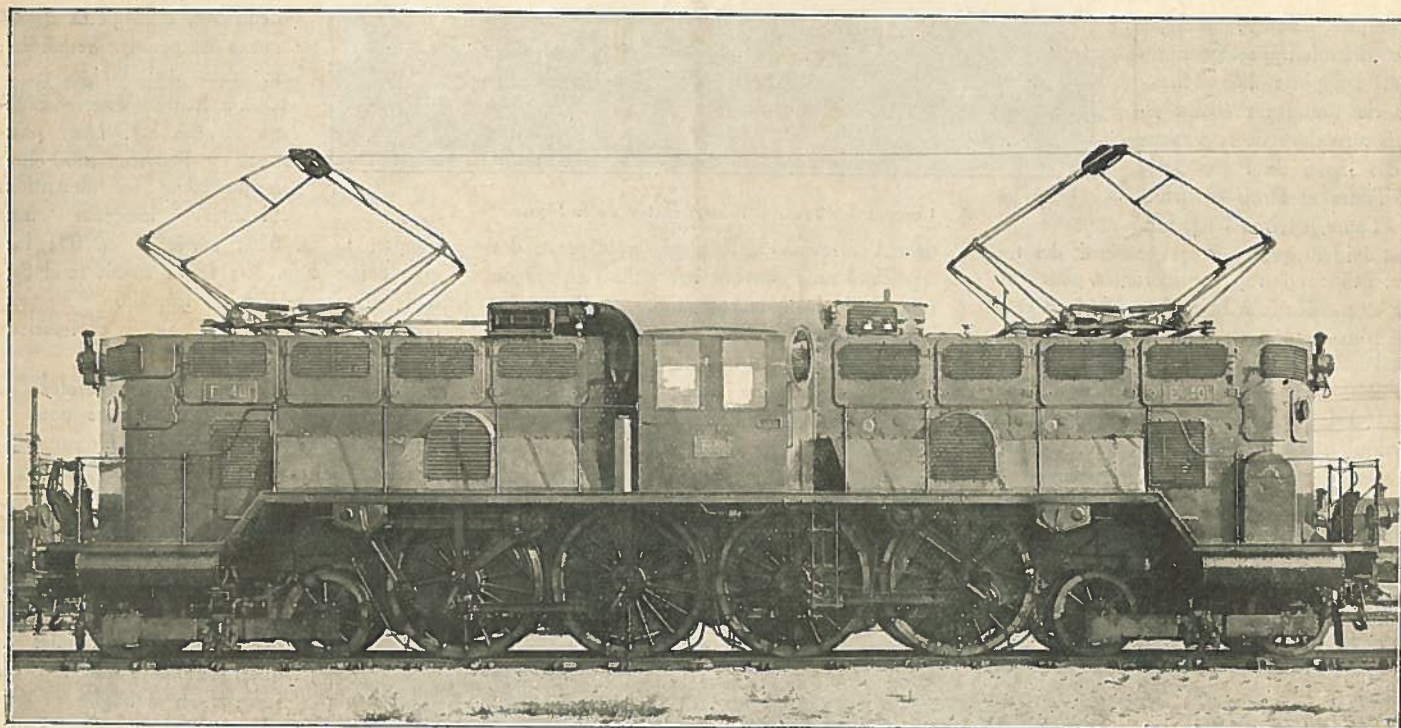
Locomotive Électrique à Grande Vitesse, Type 2 D1 Ganz
