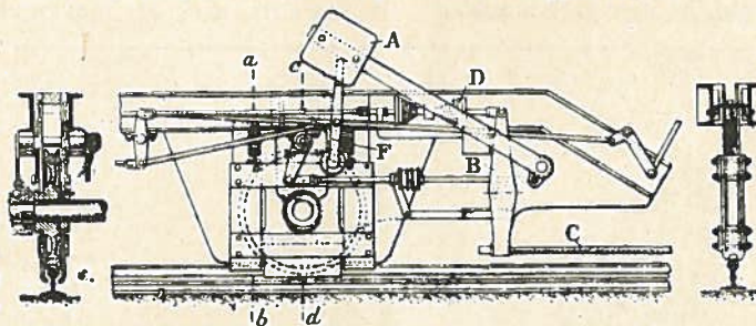
Fig. 2 Mécanisme du Frein des Wagons
