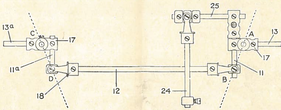
Fig. 5. — Schéma du Mécanisme de Direction
