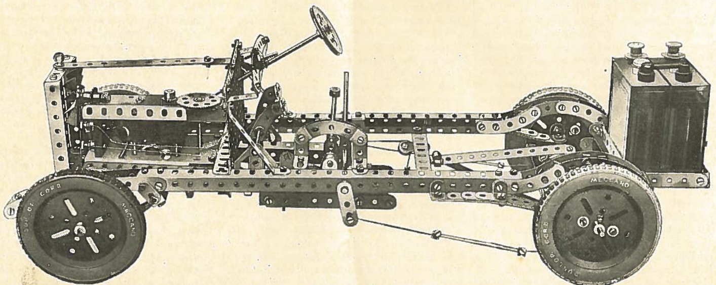
Fig. 4. — Vue générale du Châssis
