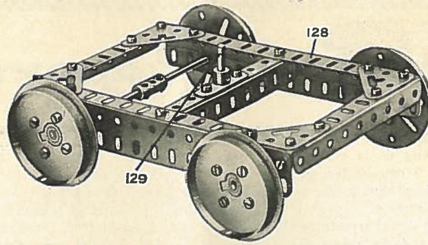
Fig. 4. — Un des deux bogies à quatre roues.
