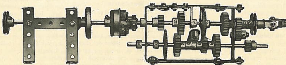
Embrayage et Boîte de Vitesses Meccano
