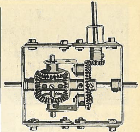
Différentiel Meccano
