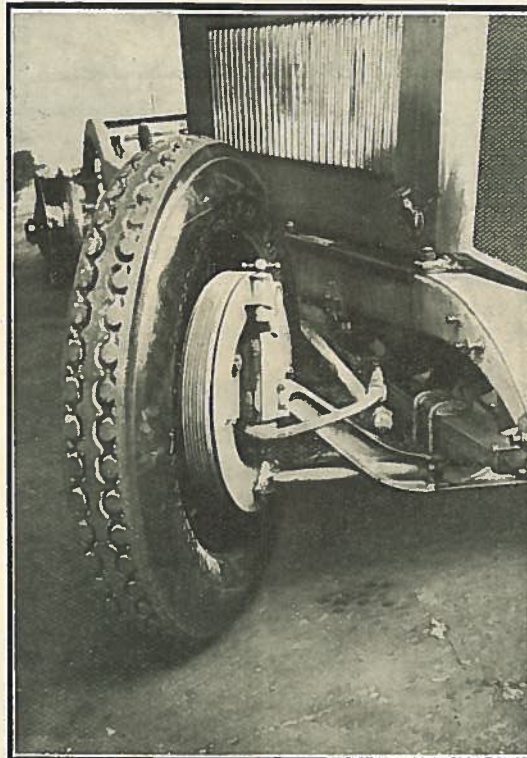
Commande de Freins avant
