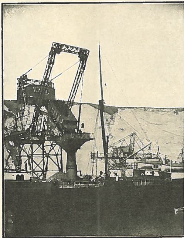
Basculeur électrique, Port de Gijon (Espagne) (Maison Demag, constr.)
