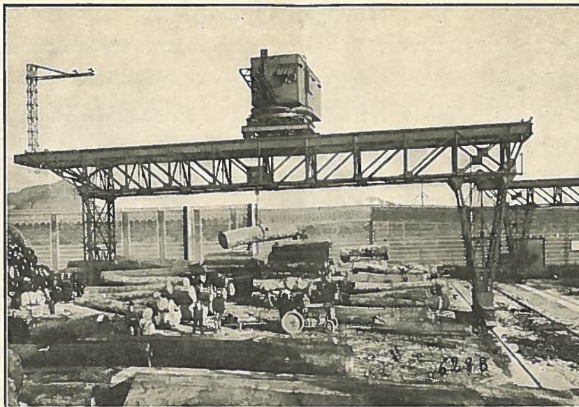
Pont Portique électrique avec chariot roulant et pivotant Puissance : 10.000 kg. Portée du crochet : 35 m. (Etab. Caillard et C ie , constr.)
