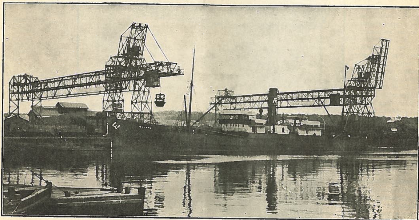
Ponts de Chargement mobiles électriques pour Houille et Minerai
