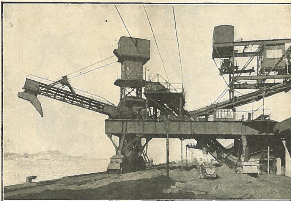
Vue d'ensemble d'un Appareil de Chargement Installation pour la manutention du Minerai de fer au port de Bone
