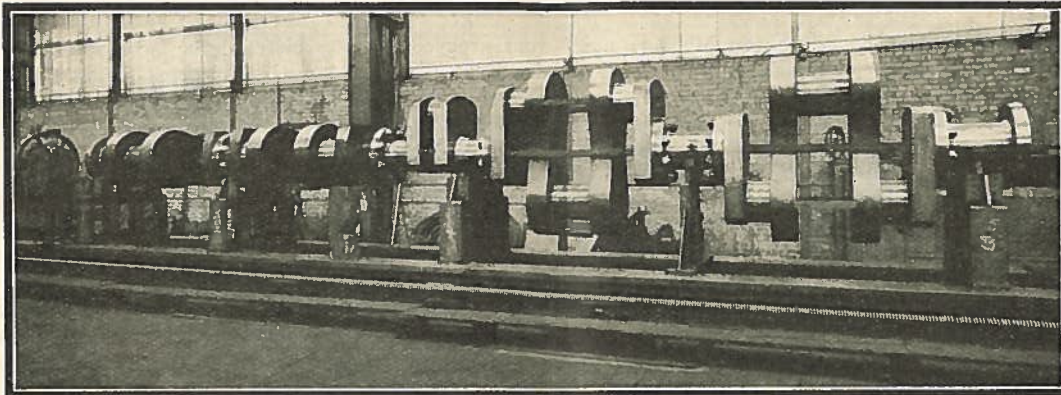
Vilebrequin de moteur Diesel
