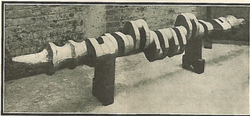
Vilebrequin d'avion fabriqué d'après la méthode d'estampage
