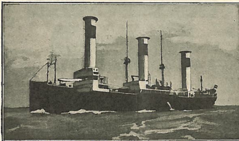
Le « Barbara », navire à Rotors, système Flettner.
