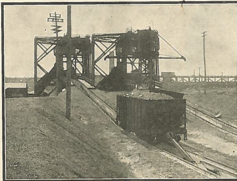
Wagon poussé par un bras mécanique vers les culbuteurs
