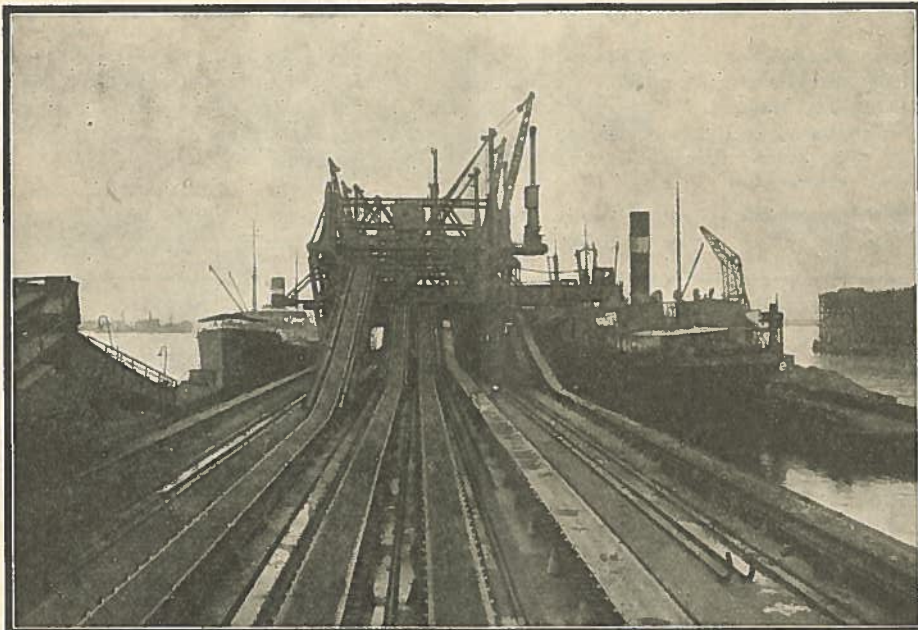
Les transporteurs à courroie amenant le charbon aux appareils.
