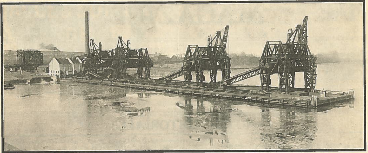
Vue générale de la jetée du port de Baltimore avec ses chargeurs de charbon.
