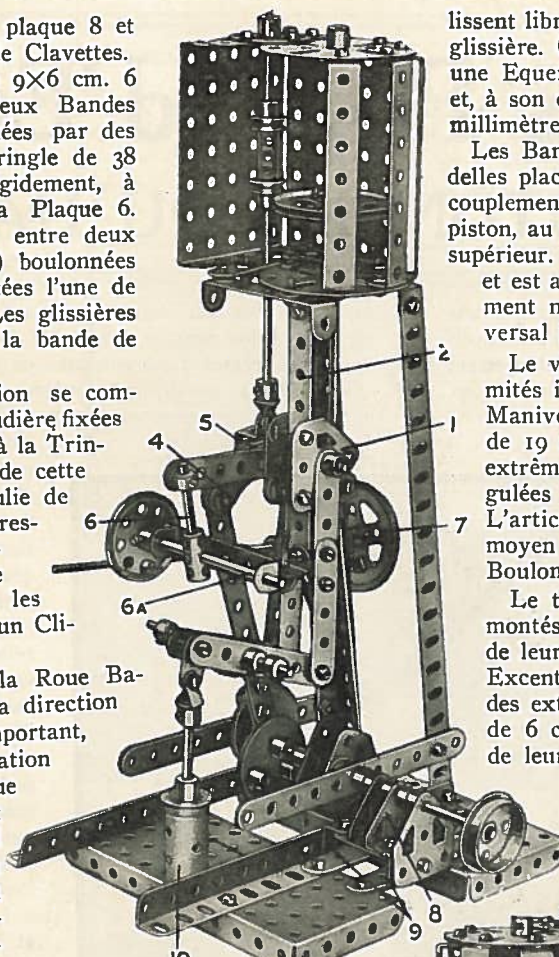
Fig. 5. La machine à vapeur verticale partiellement démontée.
