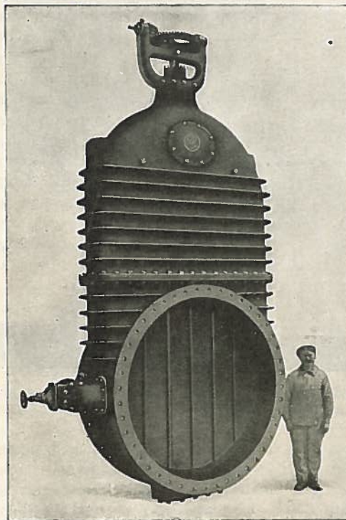
à droite: Vanne à commande hydraulique pour conduits forcés; poids 17.000 Kg.
