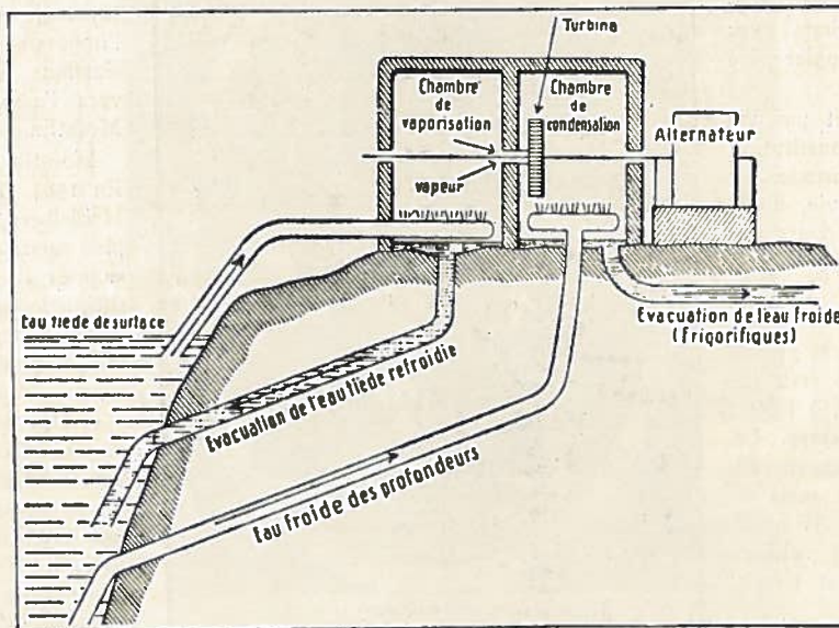
Schéma de l'installation de G. Claude
