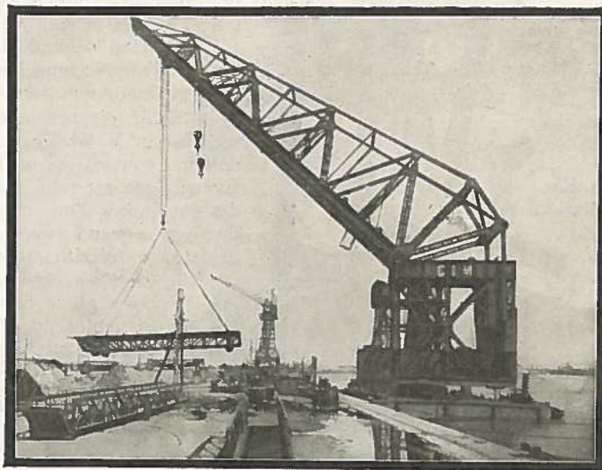
Réparation d'un Cargo sur le Dock flottant
