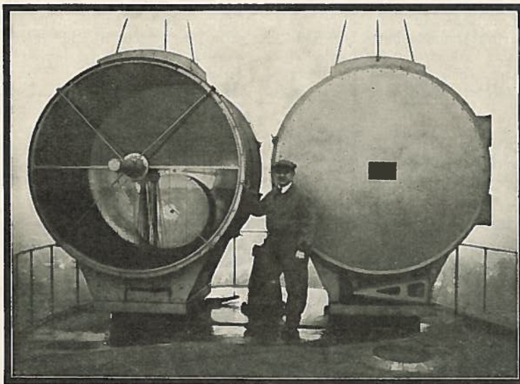
Optique du Phare du Mont-Valérien.
